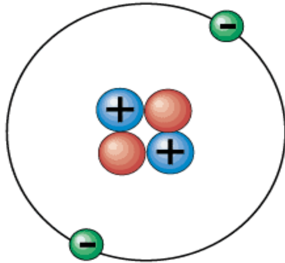
Helium atom
